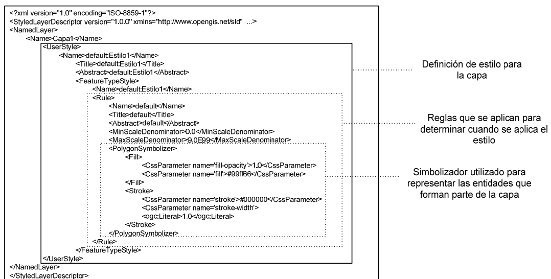
Figura 3: Ejemplo de documento SLD
