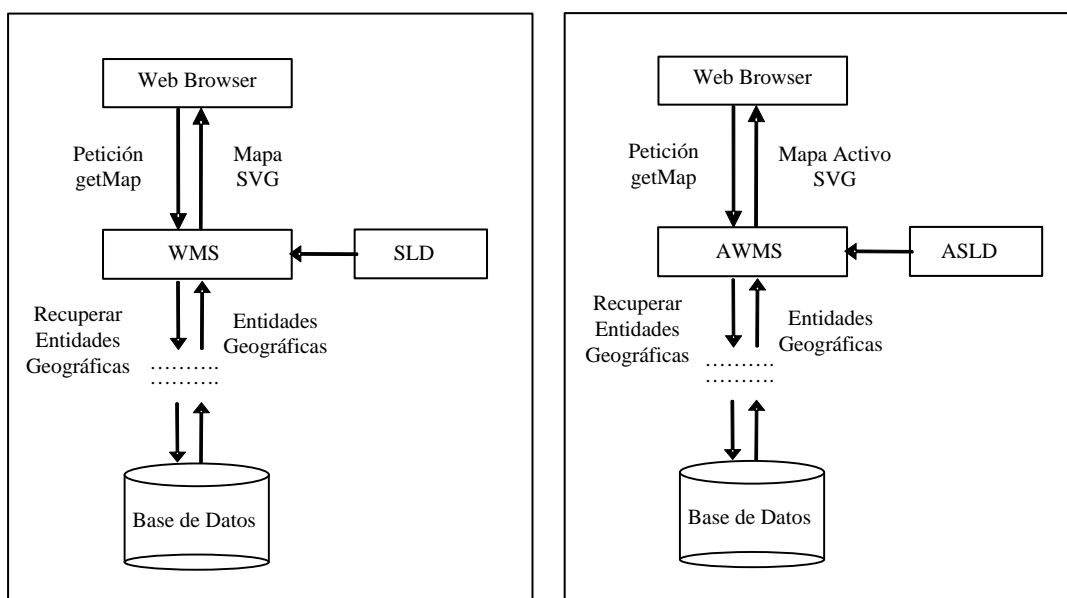
Figura 1: Arquitectura de WMS y AWMS
