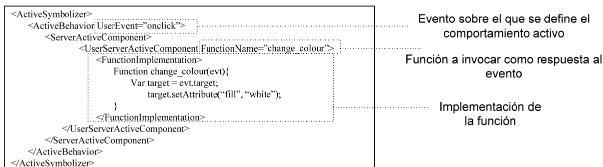
Figura 6: Ejemplo de Simbolizador Activo
