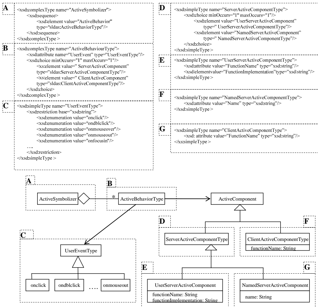
Figura 5: Descripción en XML Schema y en UML de Active Symbolizer
