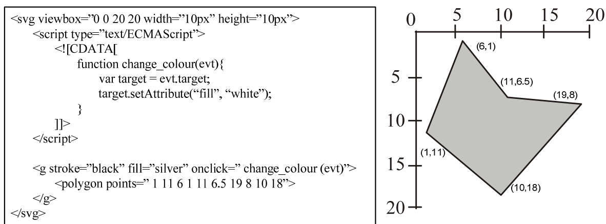
Figura 4: Mapas Activos en formato SVG
