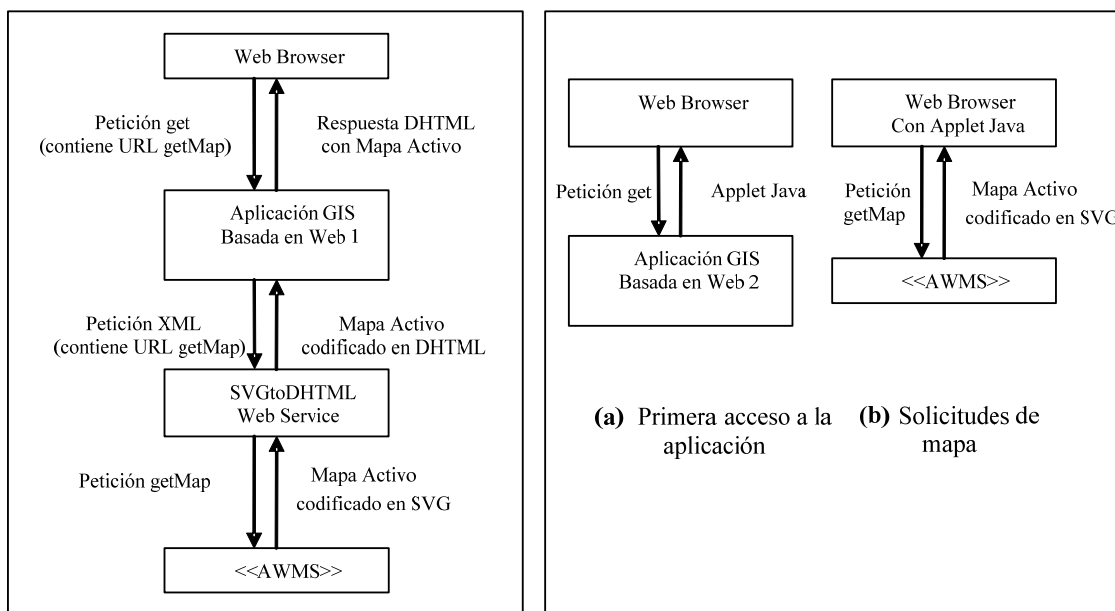
Figura 7.1: Aplicación Cliente basada en DHTML
