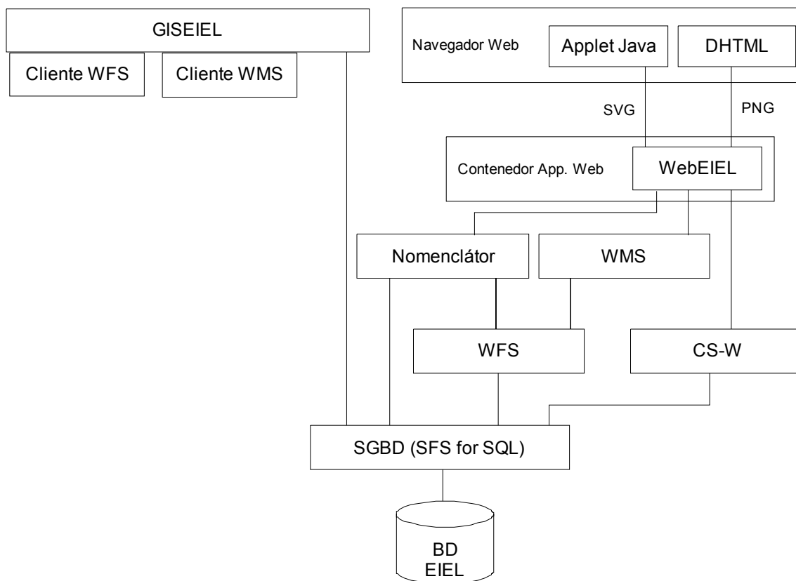
Figura 2. Arquitectura del nodo ideAC
