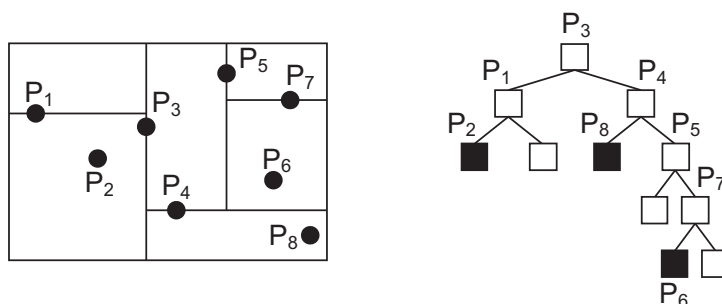
Figura 2.7: Ejemplo de construcción de un K-d-tree.
